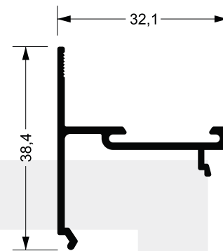
LG-077 0,324 kg/m
