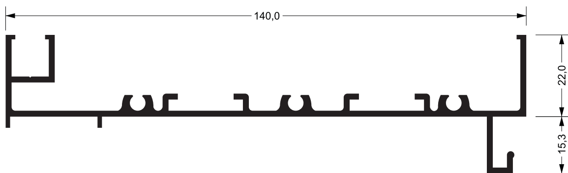
MN-001 1,314 kg/m
