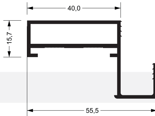
FC-293 0,651 kg/m
