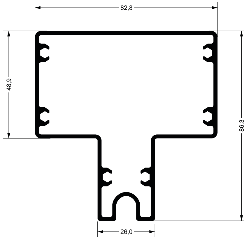
RA-223 1,978 kg/m
