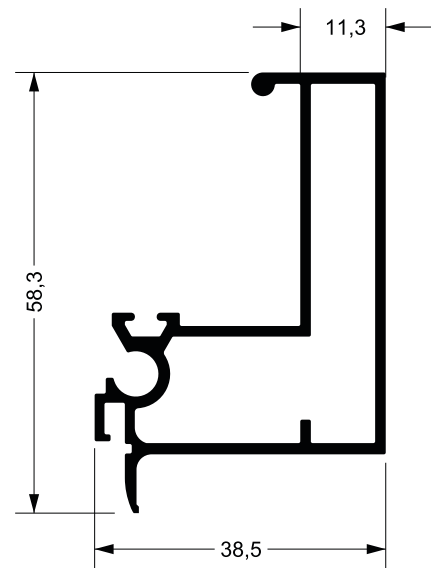
RA-256 0,800 kg/m
