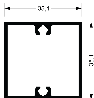
D-081 0,610 kg/m
