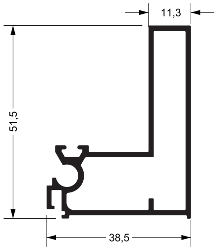
RA-245 0,742 kg/m
