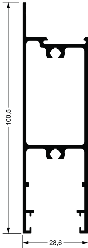
LG-007 1,200 kg/m
