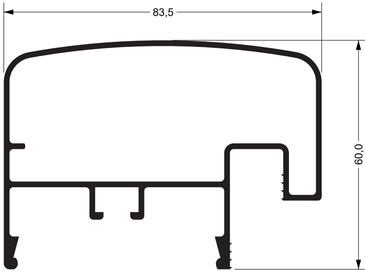
CG-083 1,321 kg/m
