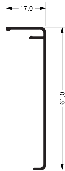
RAL-714L 0,260 kg/m
