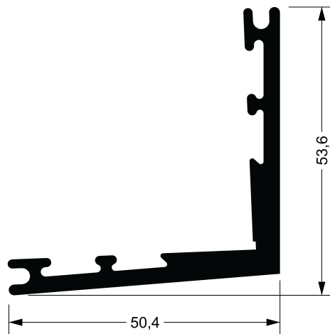
CL-006 1,047 kg/m
