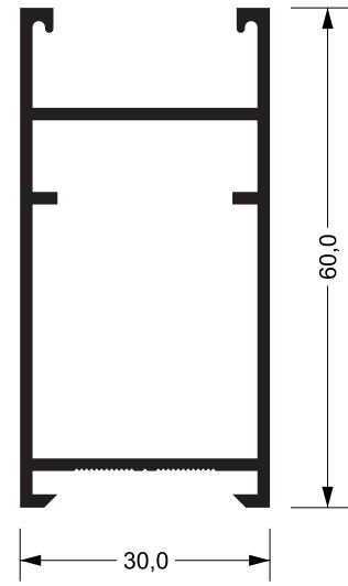
A-144 0,730 kg/m
