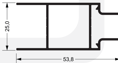
SU-191 0,455 kg/m
