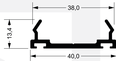
U-615 0,434 kg/m
