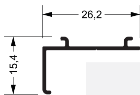
SU-084 0,126 kg/m
