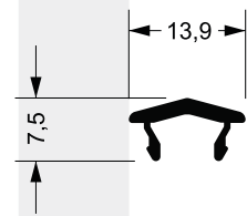
LG-111 0,127 kg/m
