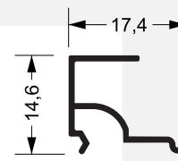
SU-202 0,733 kg/m
