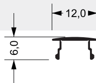
RAL-491L 0,090 kg/m
