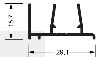
SU-008 0,244 kg/m
