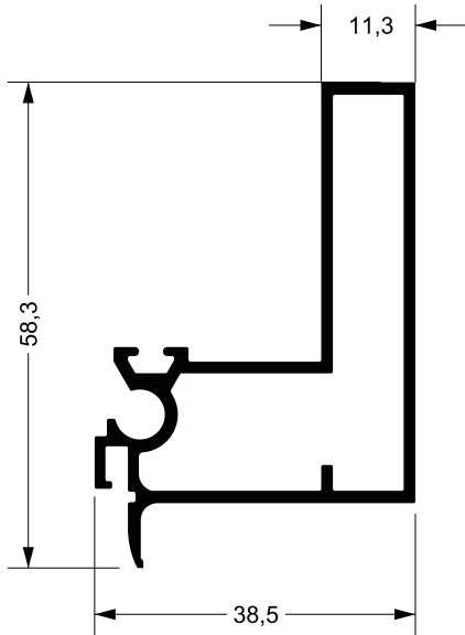
RA-255 0,765 kg/m
