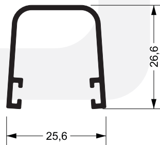
SU-107 0,271 kg/m
