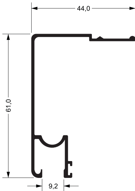
RAL-713L 0,600 kg/m
