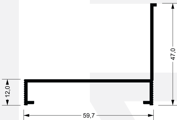
CM-173 0,509 kg/m
