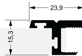
Y-343 0,284 kg/m
