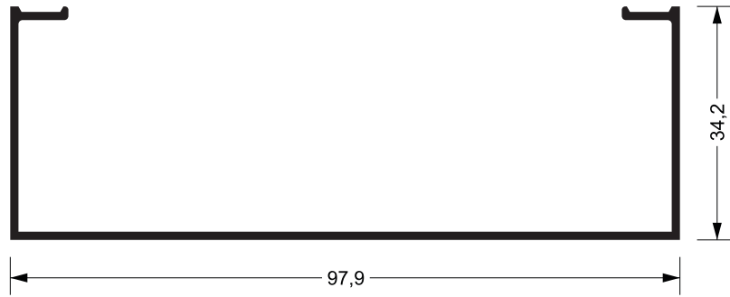
MN-050 0,734 kg/m
