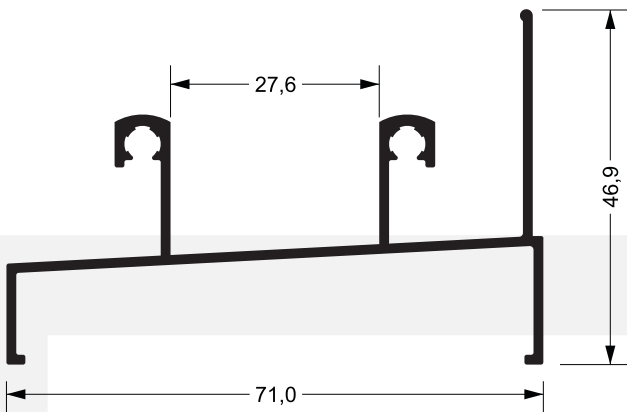
SU-002 0,691 kg/m
