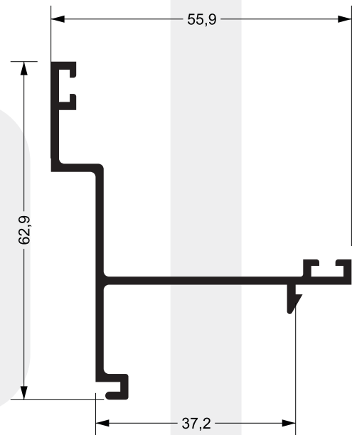
FC-249 0,604 kg/m
