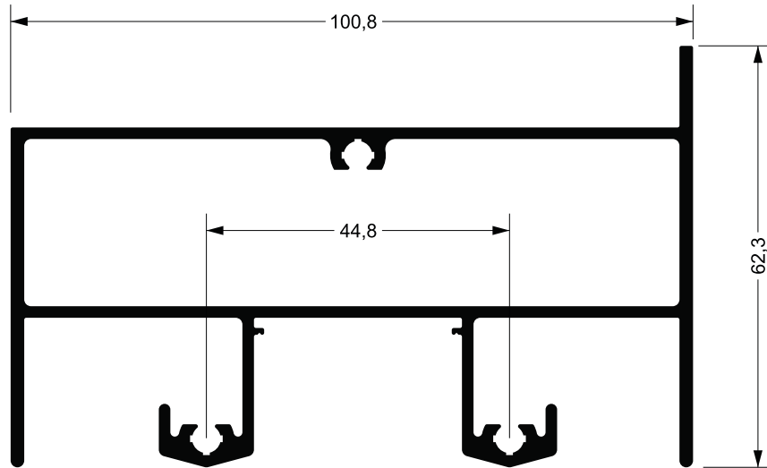
LG-004 2,019 kg/m
