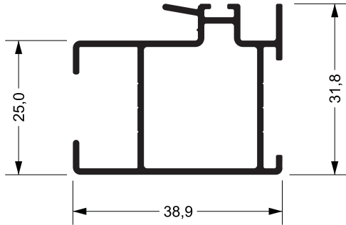
SU-056 0,560 kg/m
