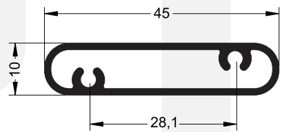
RAL-004 0,392 kg/m
