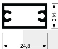
D-082 0,342 kg/m
