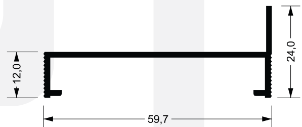
CM-174 0,409 kg/m
