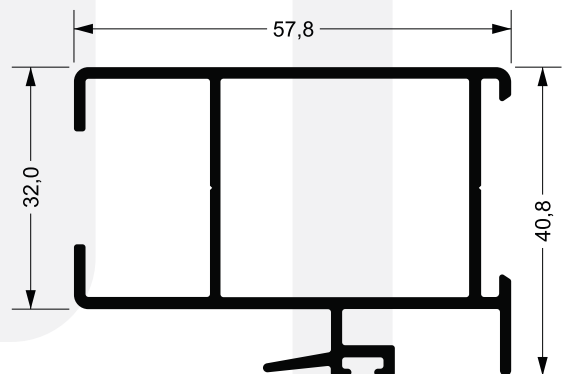
RAL-049/SB 0,872 kg/m
