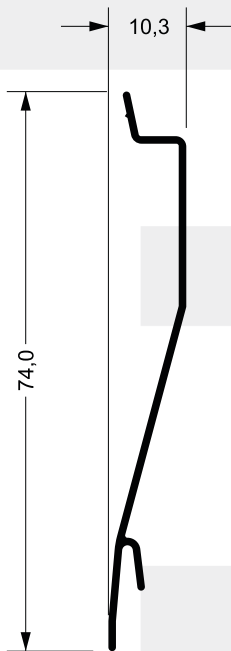
Z-201 0,275 kg/m
