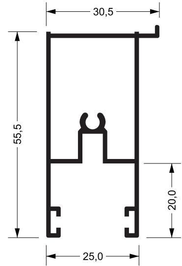
MN-007 0,707 kg/m
