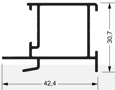
SU-040 0,470 kg/m
