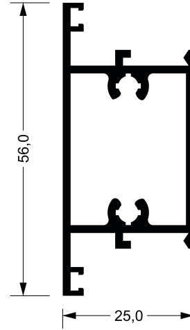
P-319 0,582 kg/m
