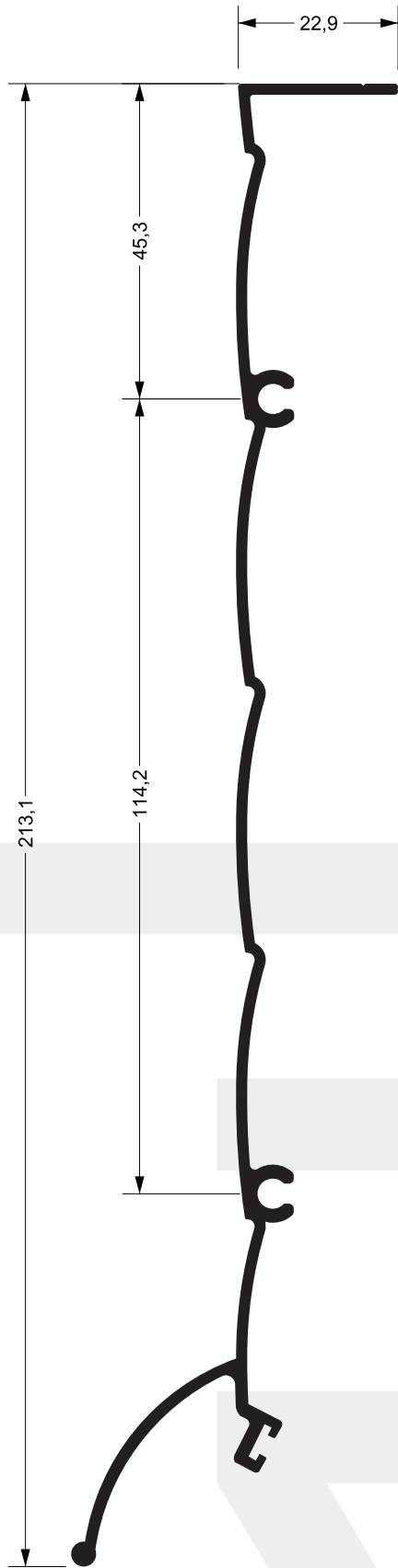
MN-039 1,356 kg/m
