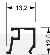
U-522 0,100 kg/m
