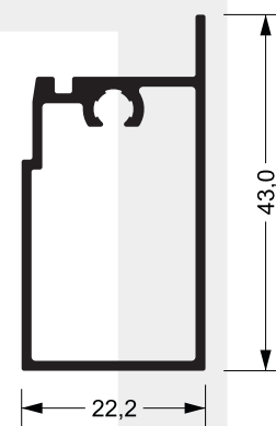
SU-073 0,447 kg/m
