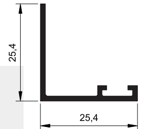
RAL-013 0,168 kg/m
