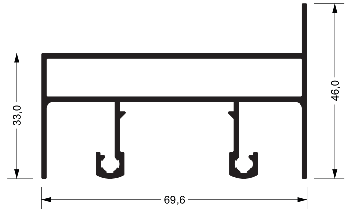
SU-006 1,086 kg/m
