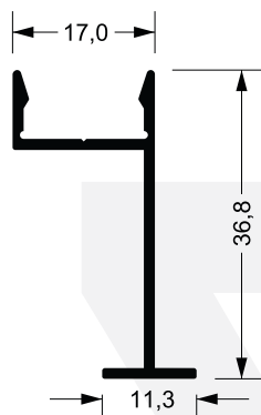
50018 0,263 kg/m
