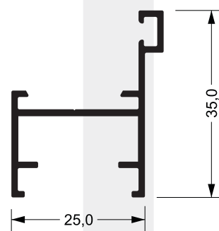
SU-079 0,352 kg/m
