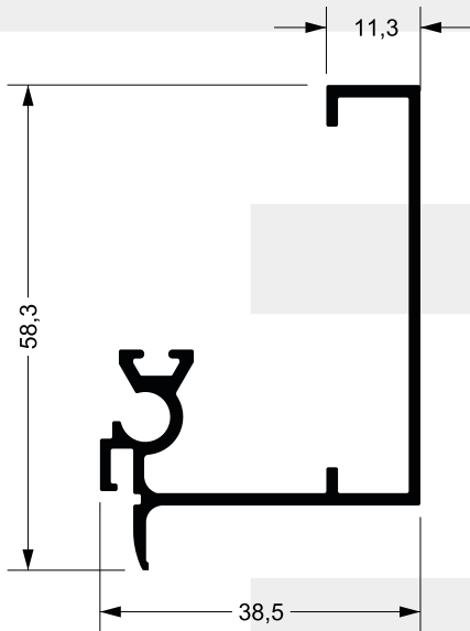
RA-258 0,590kg/m
