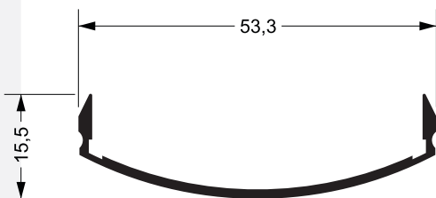
CG-074 0,242 kg/m
