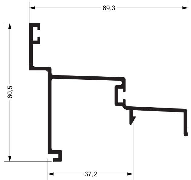
FC-222 0,759 kg/m
