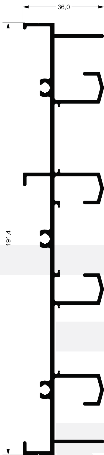
LG-070 2,075 kg/m
