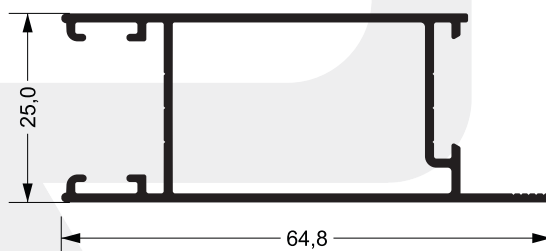
SU-245 0,597 kg/m
