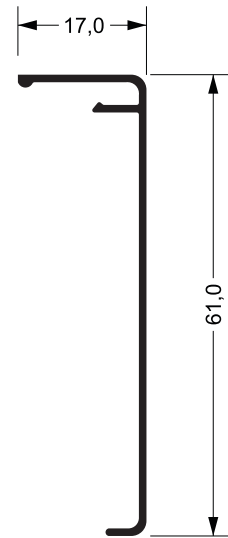
RAL-714 0,390 kg/m
