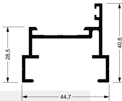
LG-056 0,652 kg/m
