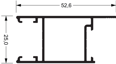
SU-039 0,575 kg/m
