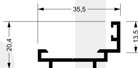
L-519 0,300 kg/m
