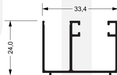
RAL-306 0,404 kg/m
