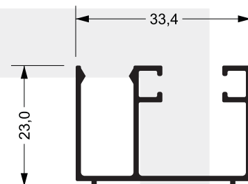
RAL-306L 0,320 kg/m
