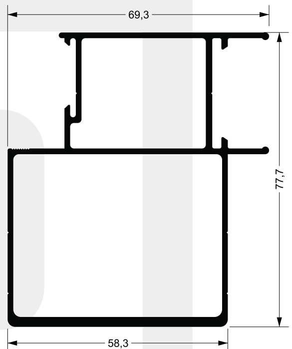
LG-054 1,575 kg/m
