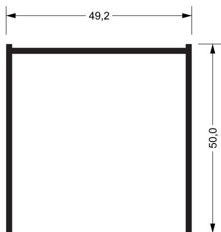
39498 0,636 kg/m
