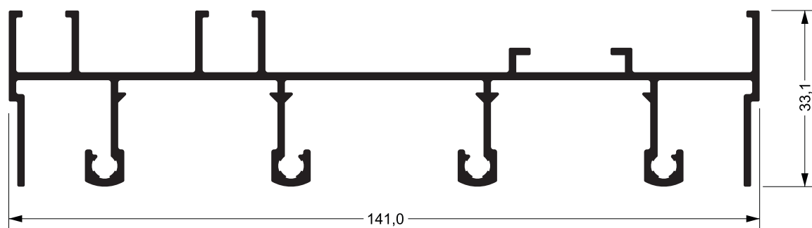
SU-121 1,461 kg/m
