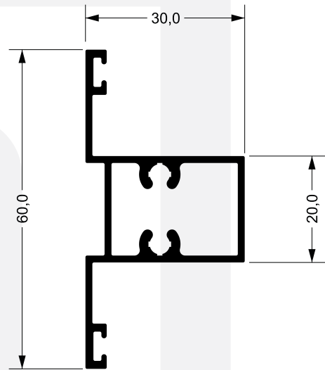
P-574 0,634 kg/m
