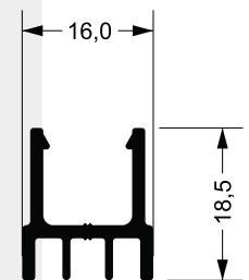
LG-157 0,251 kg/m
