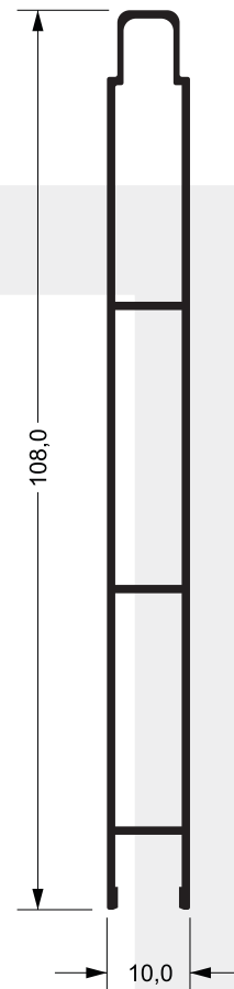
CX-185 0,841 kg/m
