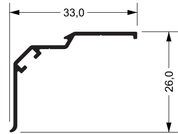
SU-276 0,168 kg/m
