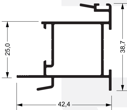
SU-042 0,545 kg/m
