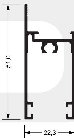
SU-053 0,489 kg/m
