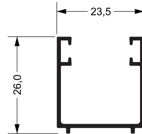
U-1108 0,360 kg/m
