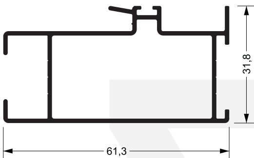
SU-239 0,734 kg/m
