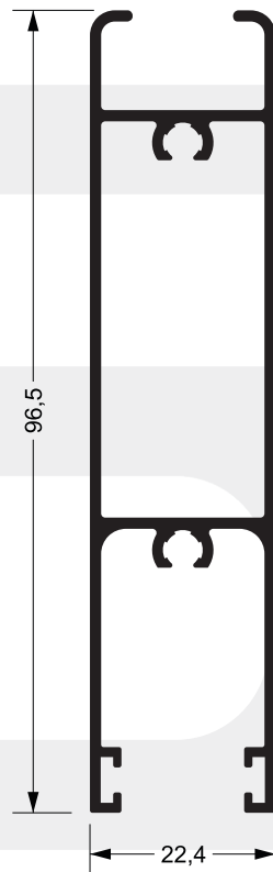
SU-226 1,014 kg/m
