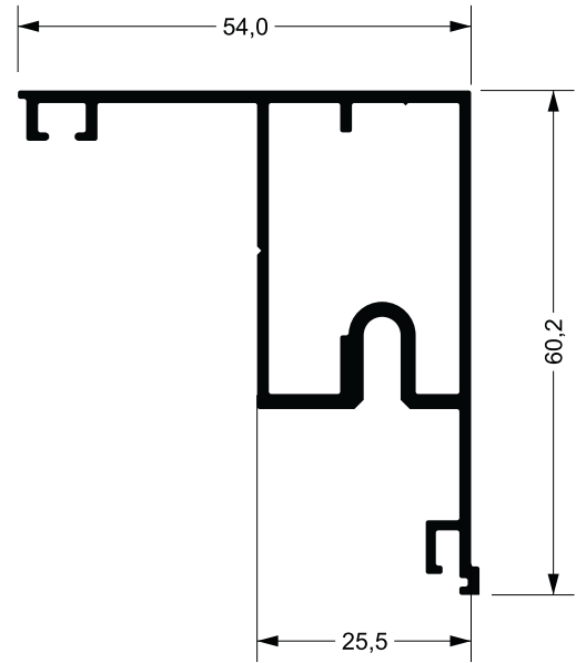
RA-516 0,894 kg/m
