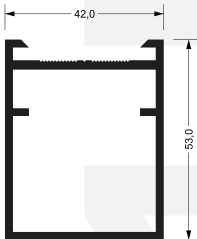
A-104 0,870 kg/m
