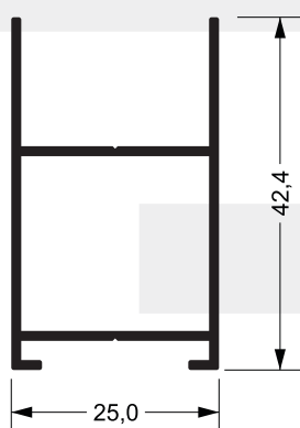
SU-072 0,439 kg/m
