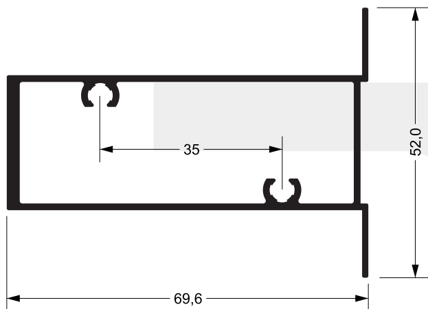
SU-009 0,980 kg/m
