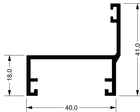
Y-181 0,570 kg/m
