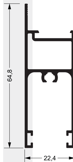
SU-246 0,642 kg/m
