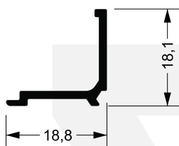
LG-015 0,142 kg/m
