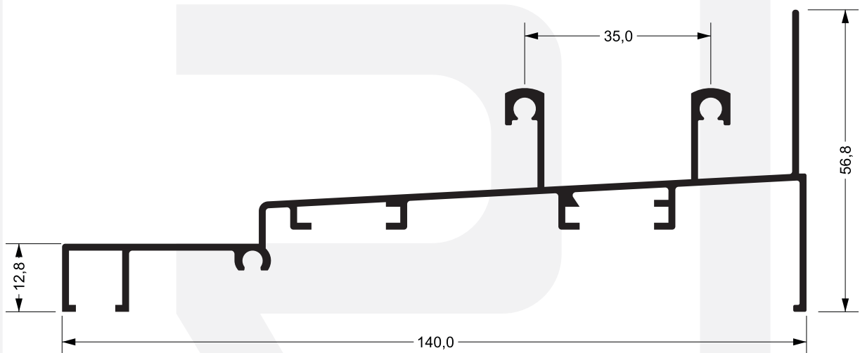
MN-010 1,420 kg/m
