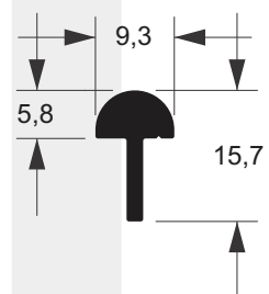
RAL-021 0,176 kg/m
