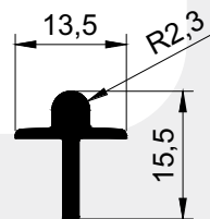
RAL-022 0,145 kg/m
