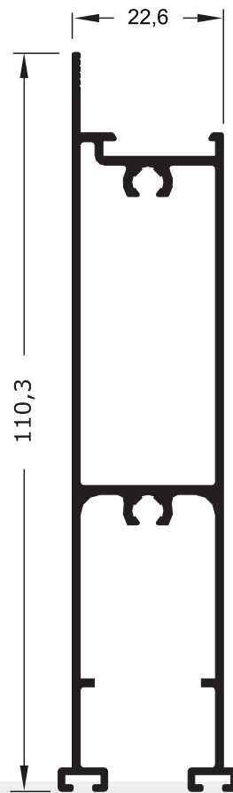
SU-225B 0,999 kg/m
