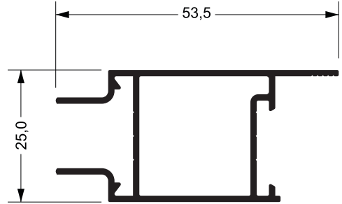
SU-192 0,492 kg/m
