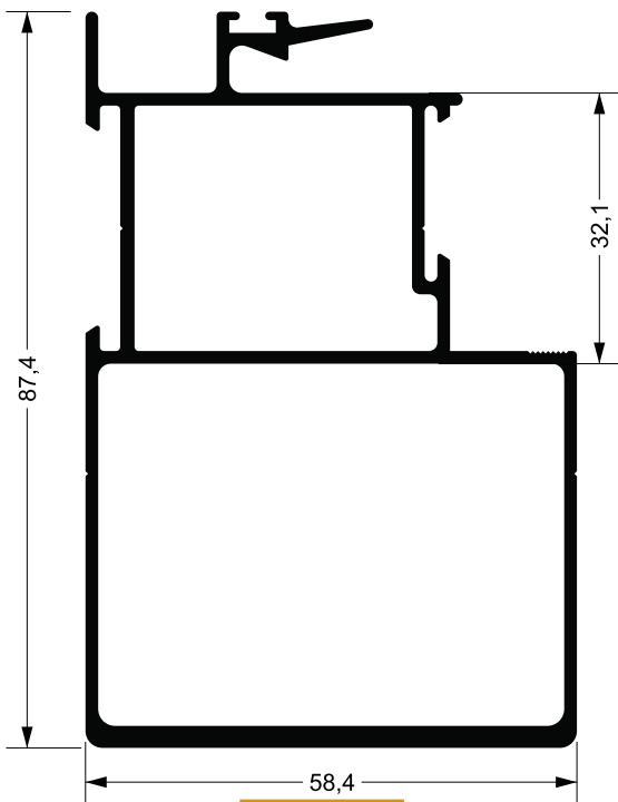
LG-052 1,675 kg/m
